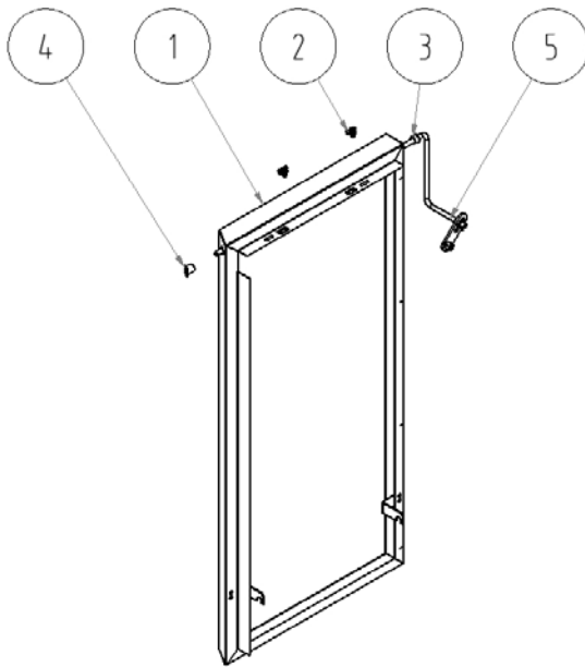
Fig. n° 14 Partie latérale gauche de la chemise
