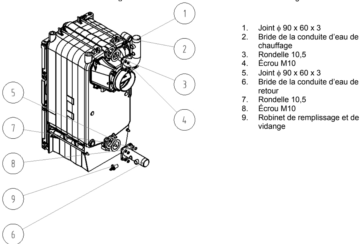
Fig. n° 11 Installation du corps de la chaudière
