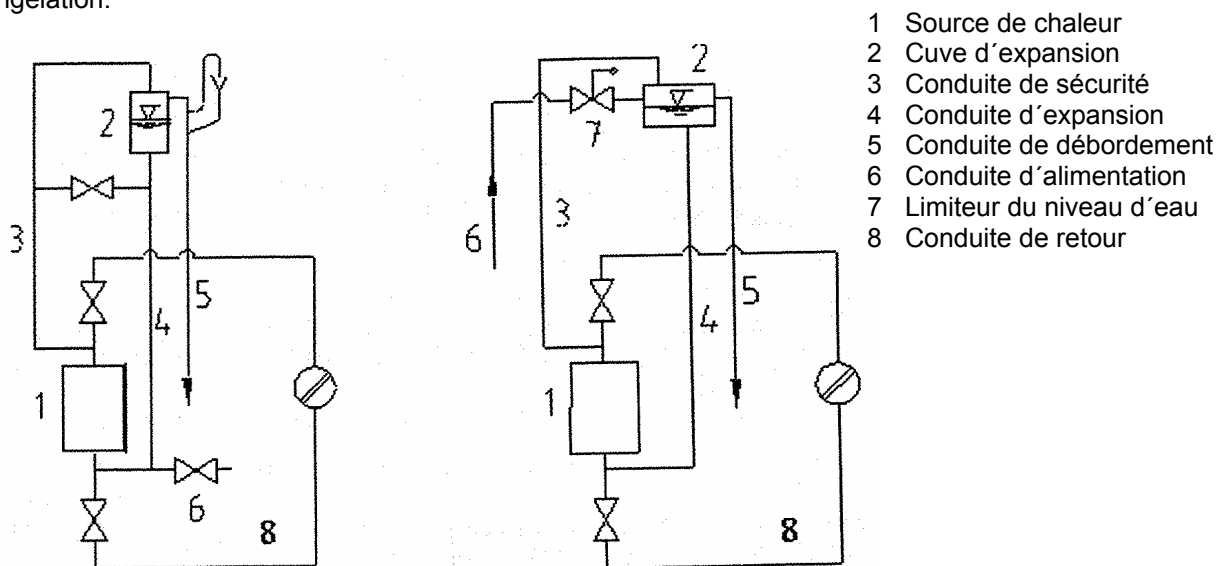
Fig. n° 7 Exemples de raccords des cuves d'expansions ouvertes
