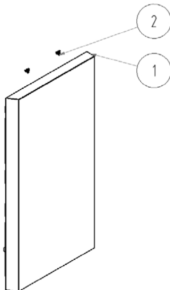
Fig. n° 13 Partie latérale droite de la chemise
