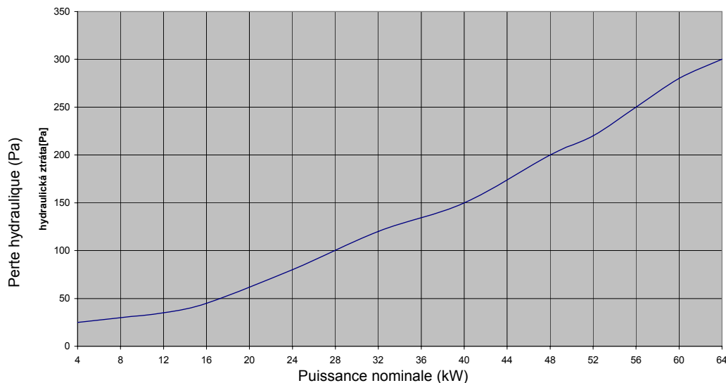
Fig. n° 1 Perte hydraulique du corps de la chaudière
