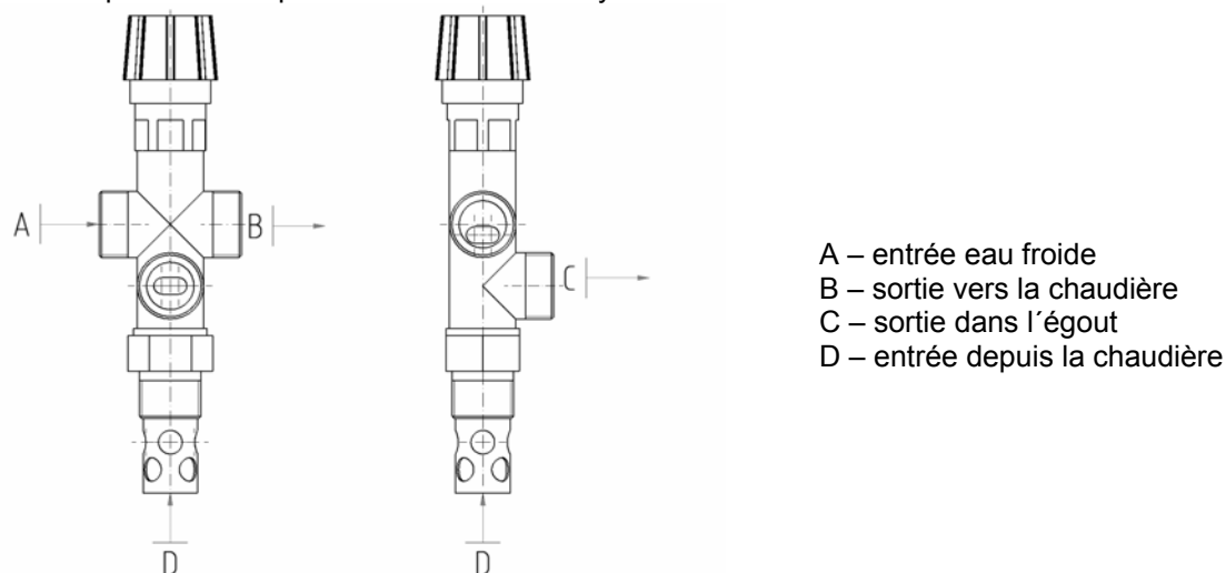
Fig. n° 5 Soupape de sécurité à deux voies DBV 1 - 02
