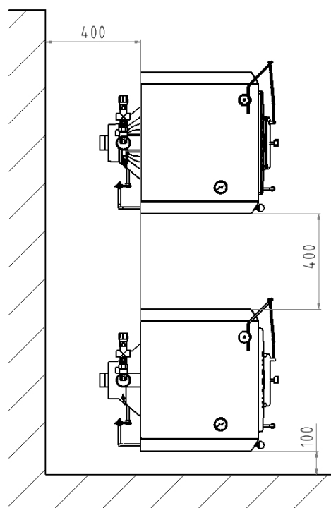
Fig. n° 9 Disposition des chaudières dans la chambre de chauffe
