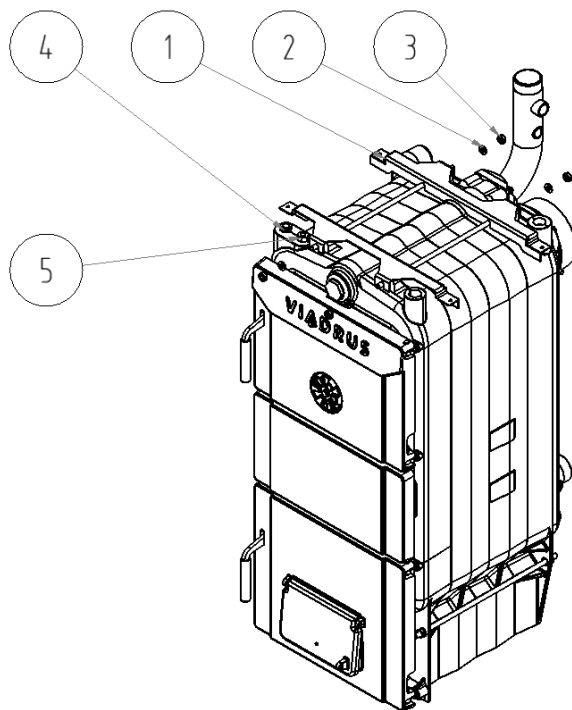
Fig. n° 12 Montage des consoles de chemise
