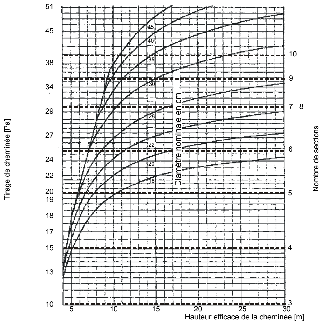
Fig. n° 2 Détermination de la diamètre de cheminée
