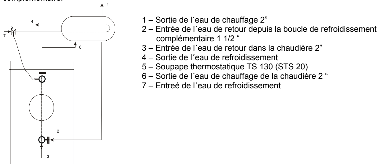
Fig. n° 4 Schéma hydraulique de raccordement de la boucle de refroidissement
