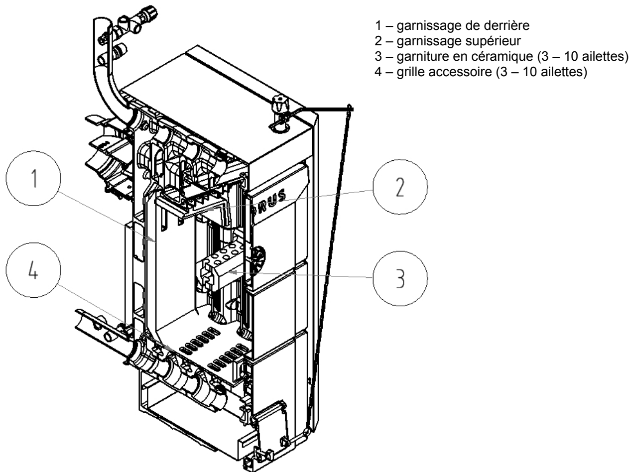
Fig. n° 3c) Combinaison de la chaudière VIADRUS HERCULES U 26 – installation de l'équipement accessoire
