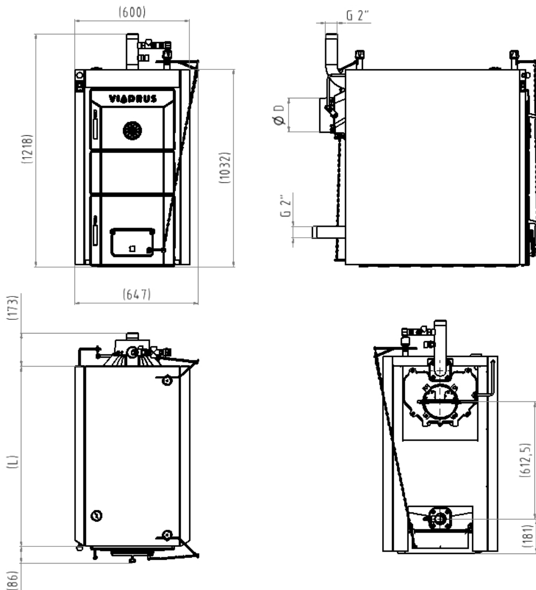
Fig. n° 10b) Dimensions d'installation de la chaudière VIADRUS HERCULES U 26 à 8 – 10 ailettes
