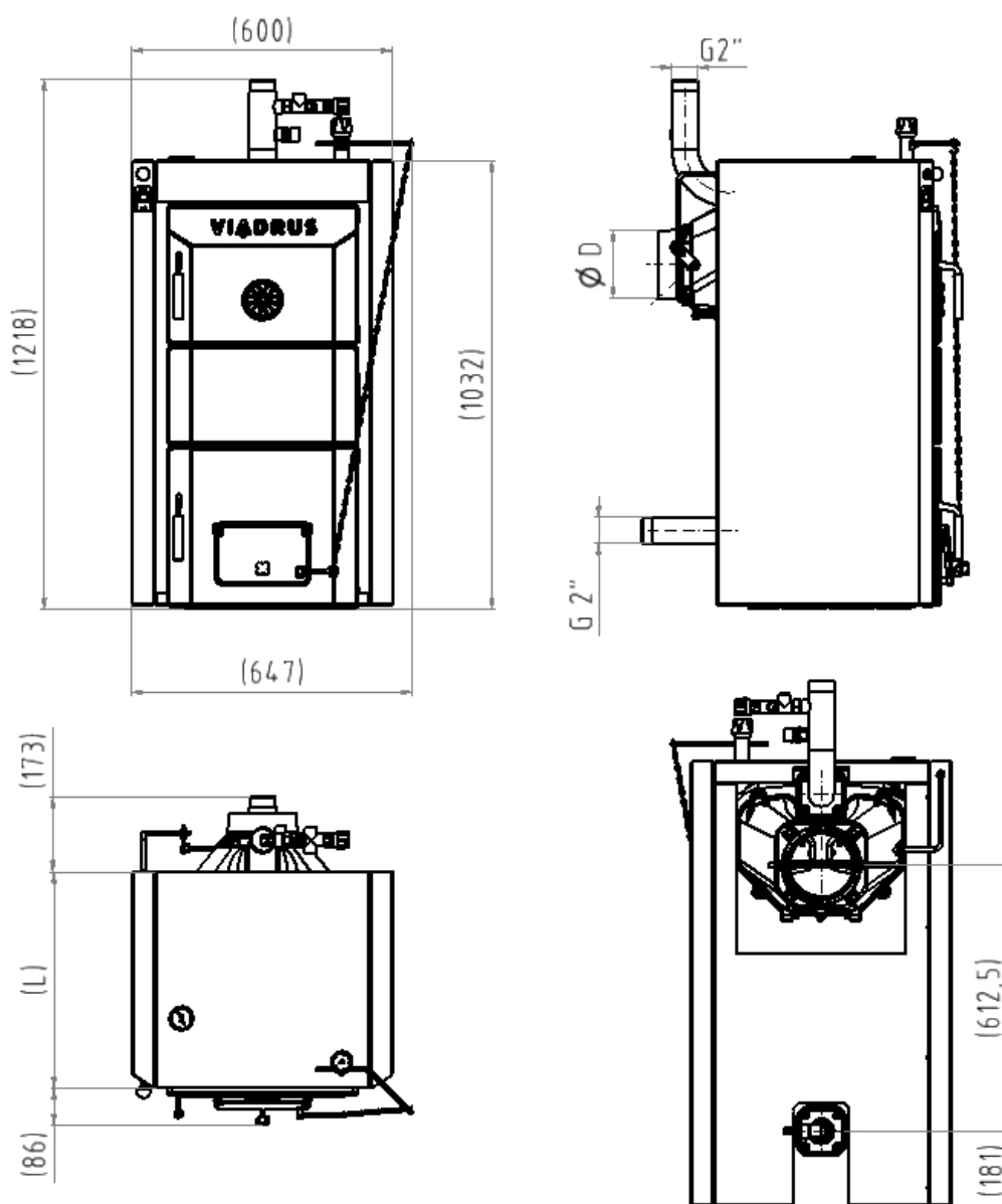
Fig. n° 10a) Dimensions d'installation de la chaudière VIADRUS HERCULES U 26 à 3 – 7 ailettes
